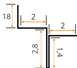
Tabica Pré-pintada 40 x 48
