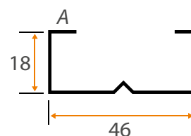
Canaleta C (F530)
